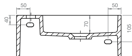
SECCIÓN A-A
